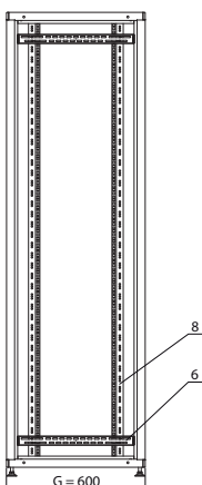
Вид с боку (шкаф глубиной 600 mm)
