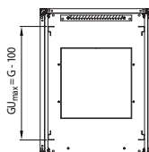
Разрез C-C (шкаф глубиной 800 mm)
