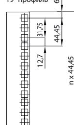
Монтажный 19" профиль
