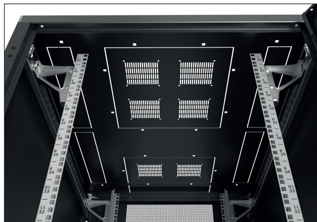
Вид верхней плиты шкафа SZB IT
