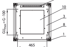
Разрез C-C (шкаф глубиной 600 mm)
