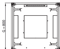
Разрез D-D (шкаф глубиной 800 mm)
