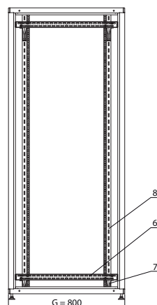
Вид с боку (шкаф глубиной 800 mm)
