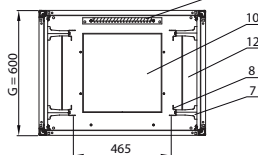
Разрез D-D (шкаф глубиной 600 mm)
